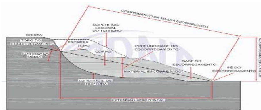
Figura 7: Esquema da instabilidade geotécnica Fonte: https://qualidadeonline.wordpress.com/2013/02 .
