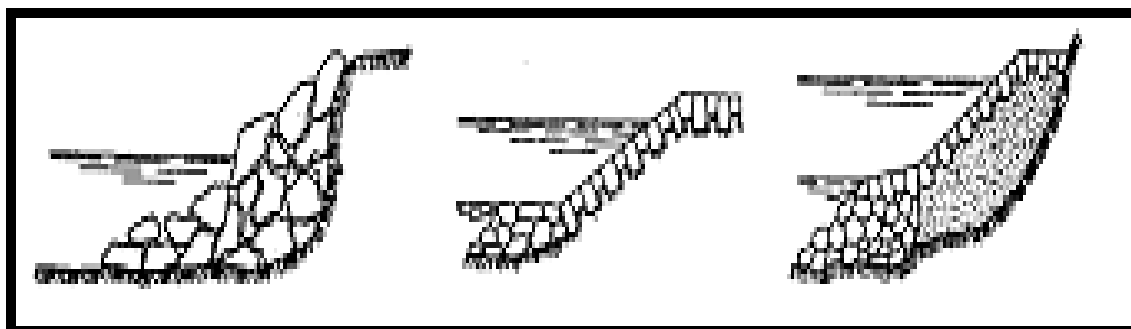
Figura 10: Tipos de proteção por enrocamento. Fonte: Martins, 2001.
