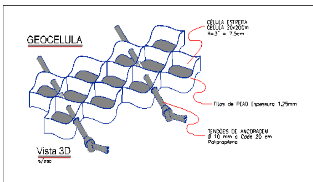
Figura 9: Detalhe da Geocelula Fonte: DNIT - 2012
