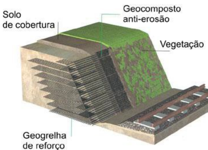
Figura 8: Detalhe de reforço com geogrelha Fonte: Antunes, 2008.
