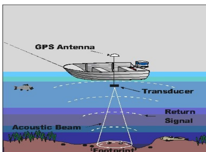
Figura 11: Sonar fazendo levantamento batimétrico. Fonte: www.mundogeo.com , 2014.
